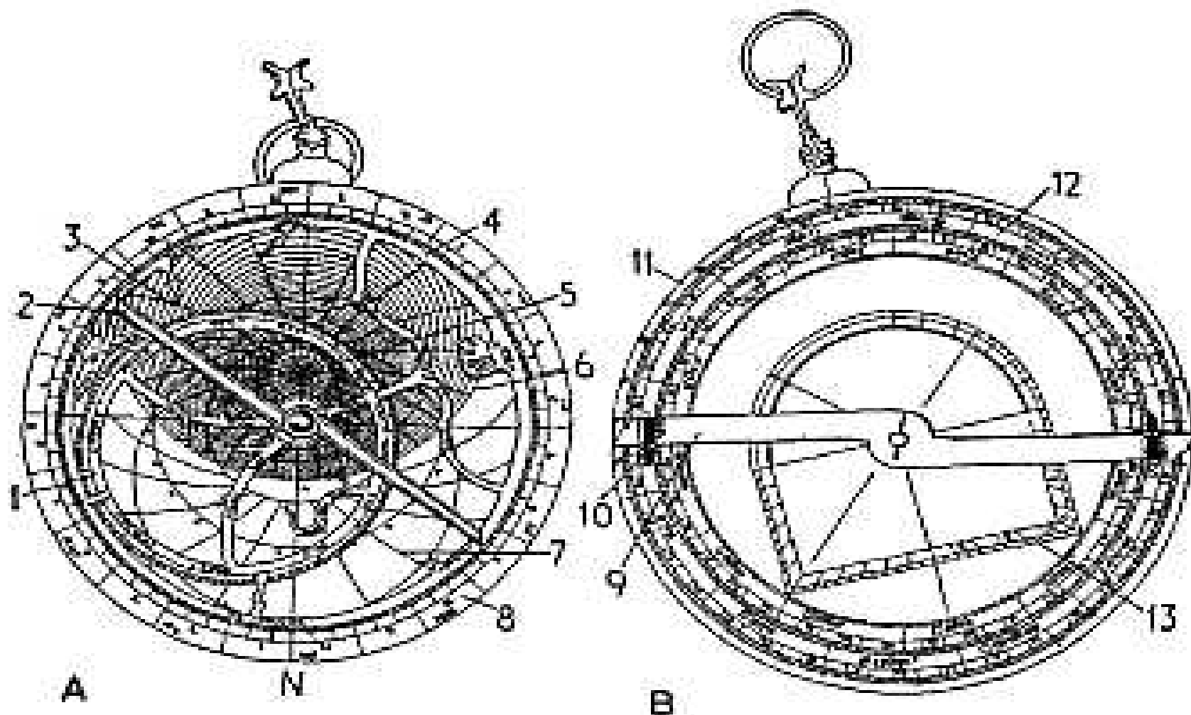
ASTROLABE: A. FRONT. B. BACK
